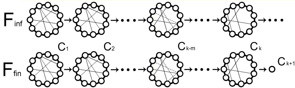
Рис. 1. Бесконечный фрейм F_{inf} и конечный фрейм F_{fin}
