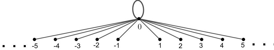
Рис. 1. Счетный граф G с множеством вершин \mathbb{Z} , все вершины связаны только с 0.
