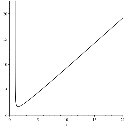
Рис. 2. График функции \lambda_3(x) .
