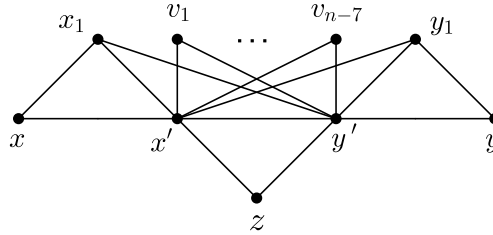
FIG. 1. Graph F_n^1
